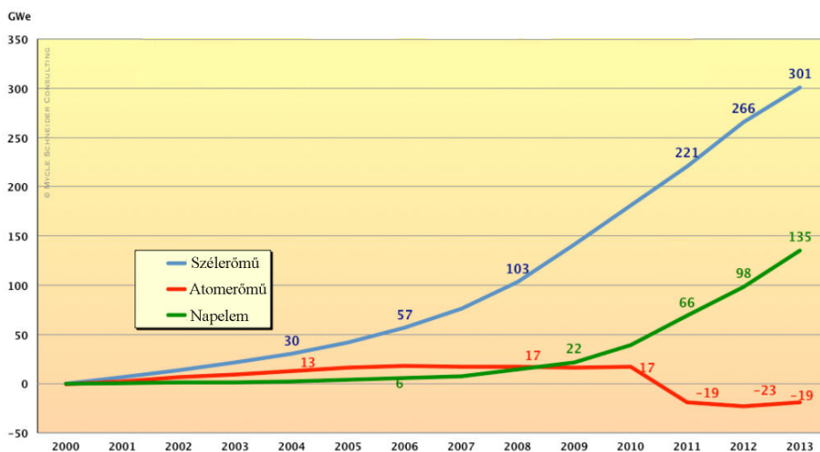
3. ábra: A villamos hálózatba integrált szél- nap- és atomenergetikai kapacitások változása a 2000. évi állapothoz képest, globális kitekintésben [16]
